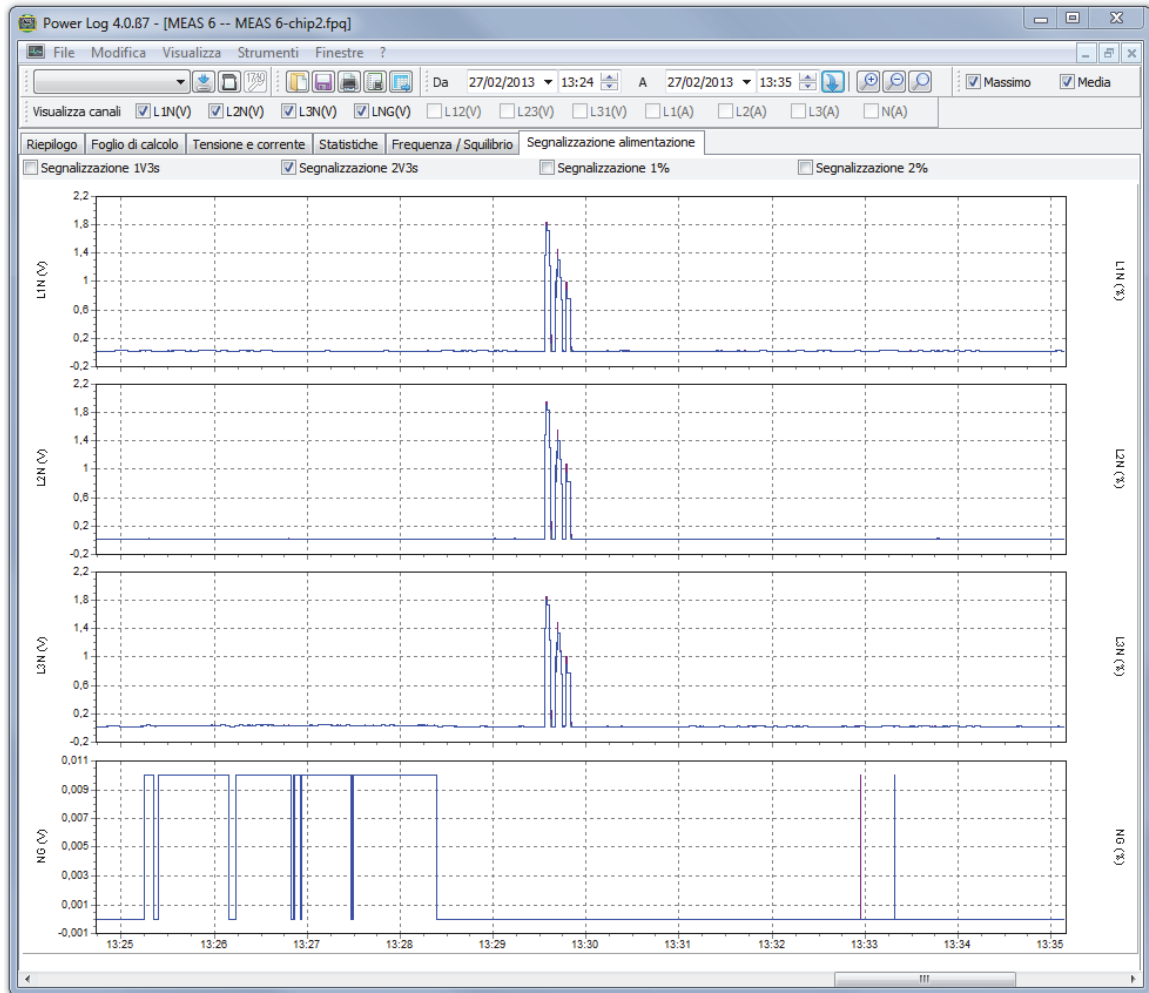
Figura 18. Forme d'onda di segnalazione alimentazione
