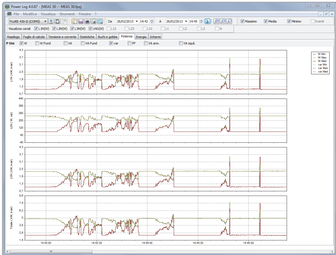
Figura 11. Grafico dei dati in funzione del tempo con potenza attiva e reattiva selezionate
