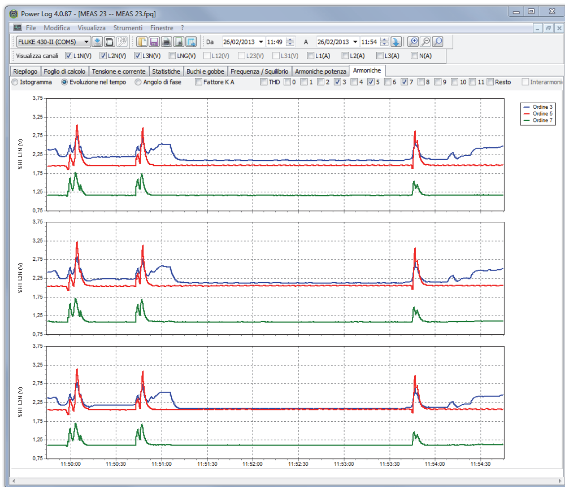
Figura 7. Evoluzione nel tempo delle armoniche con i canali selezionati
