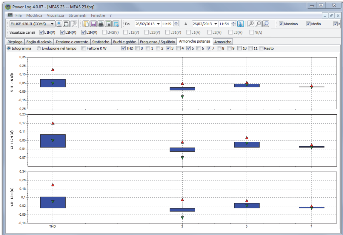
Figura 17. Armoniche potenza
