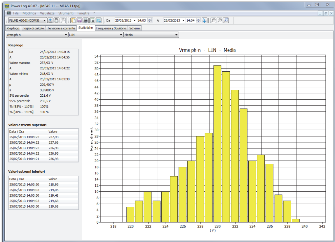
Figura 6. Statistiche con il canale A selezionato
