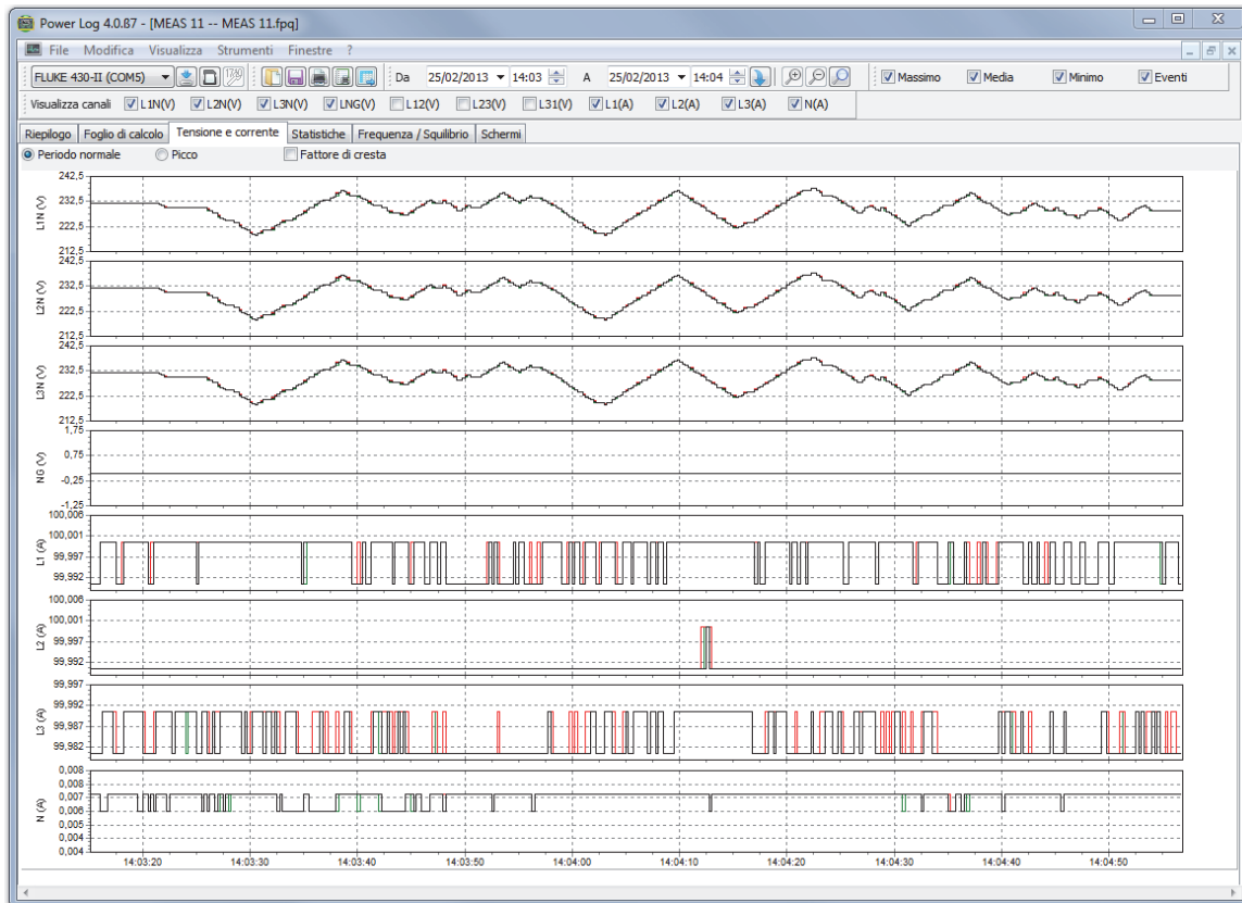
Figura 5. Grafico dei dati di tensione e corrente in funzione del tempo con i canali selezionati visibili
