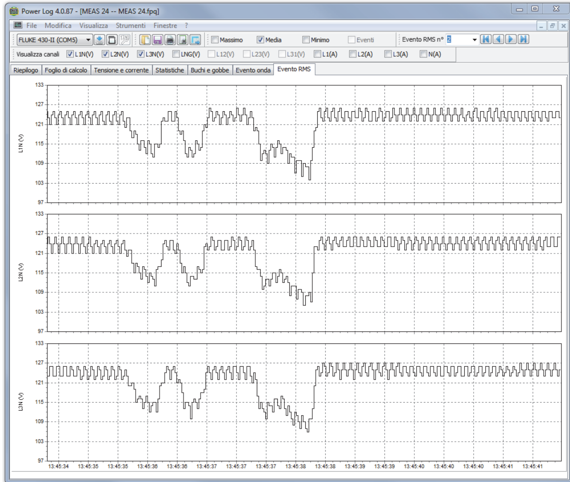
Figura 16. Profili eventi
