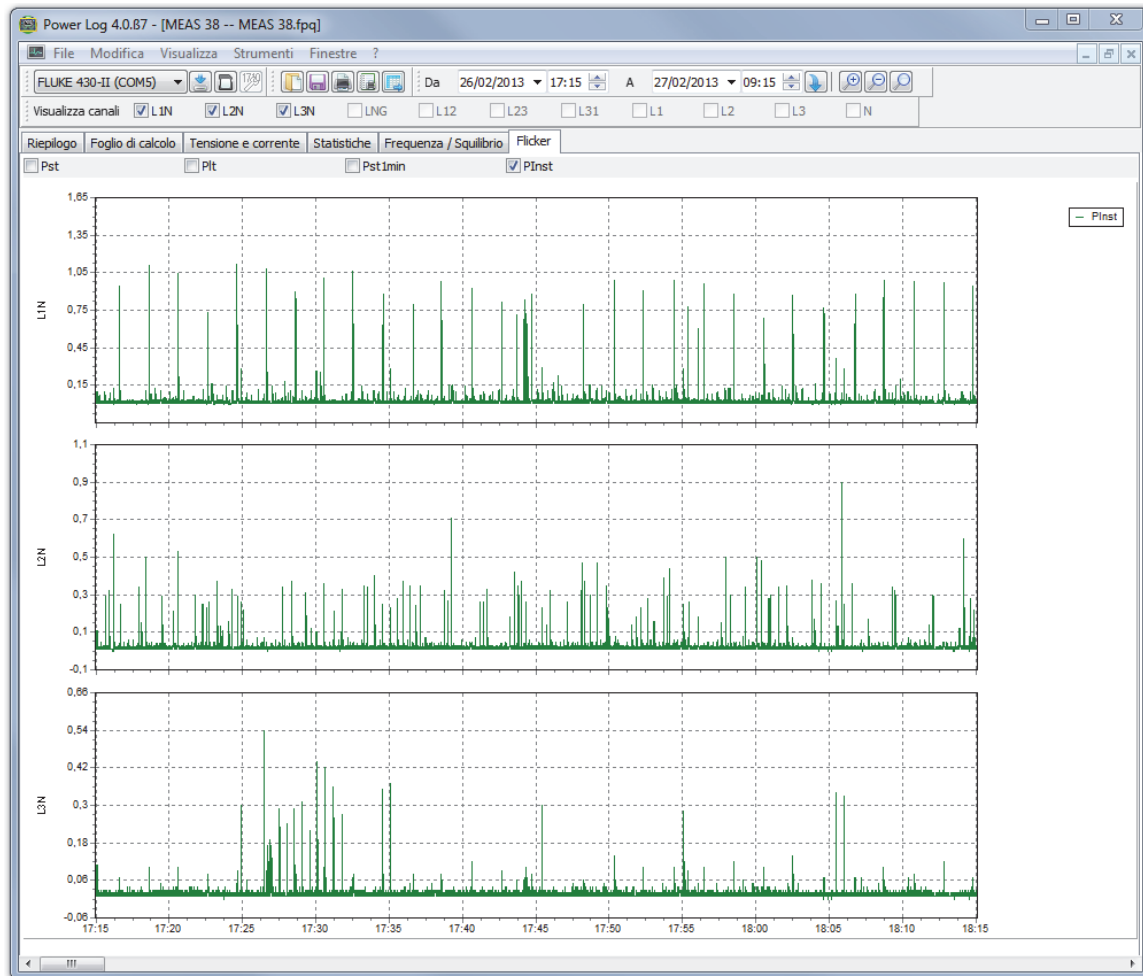
Figura 13. Forme d'onda di flicker
