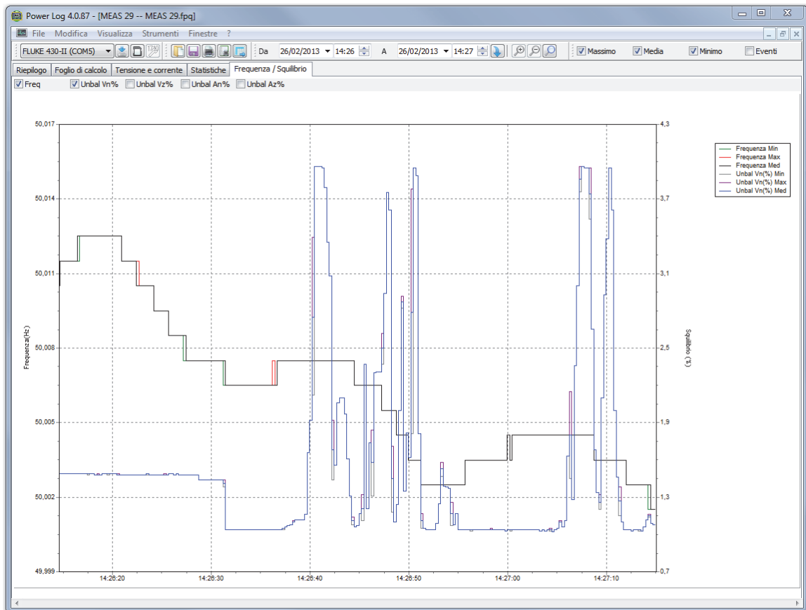
Figura 10. Grafico dei dati in funzione del tempo per Frequenza/Squilibrio - Frequenza visualizzata
