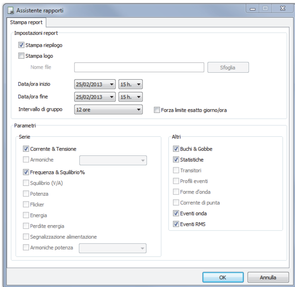
Figura 19. Opzioni della finestra Assistente rapporti
