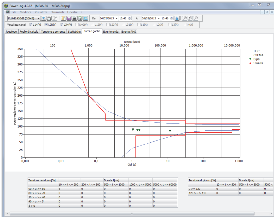
Figura 9. Buchi e gobbe
